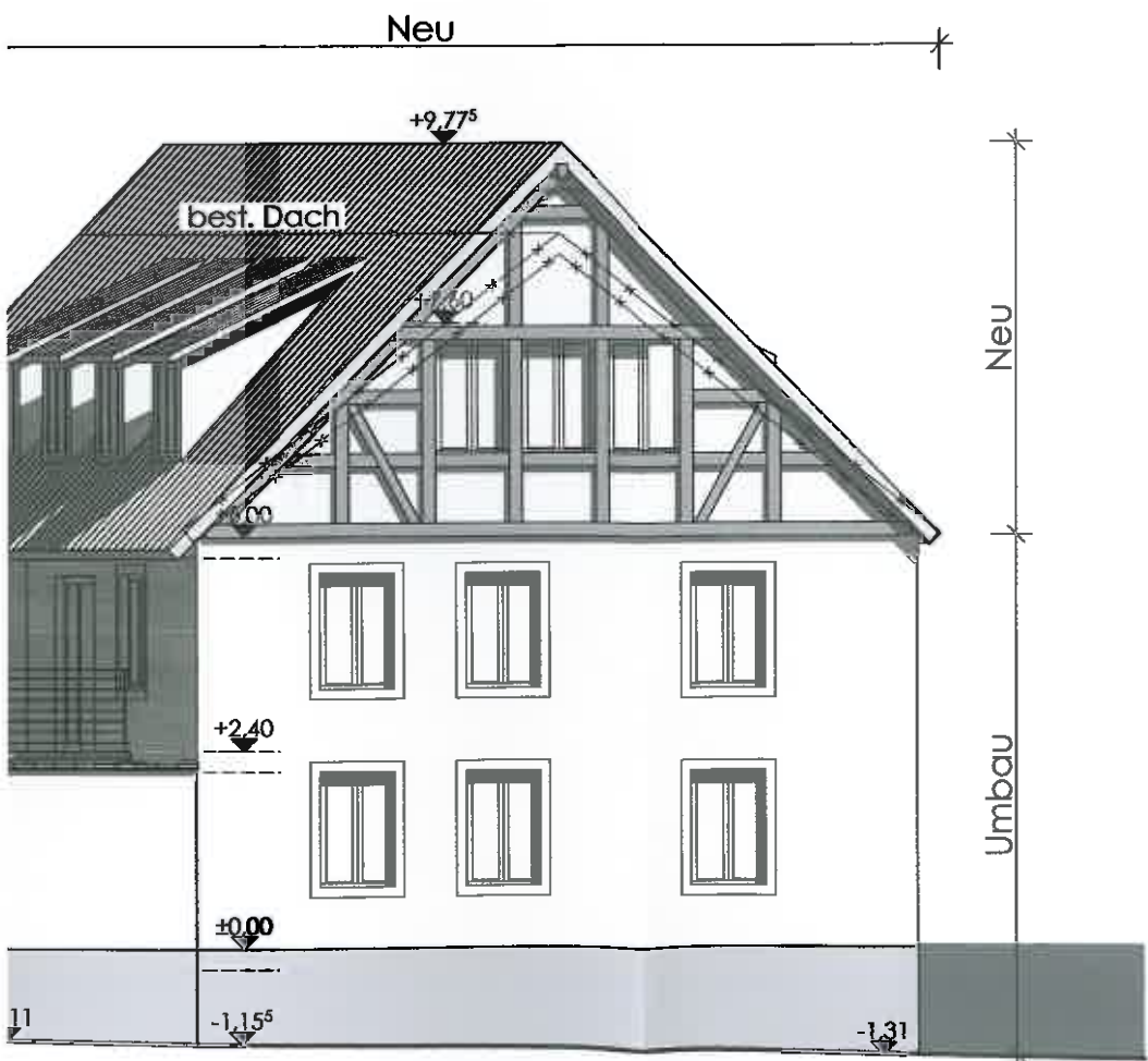
Ostansicht - Würzburger Straße Neu
