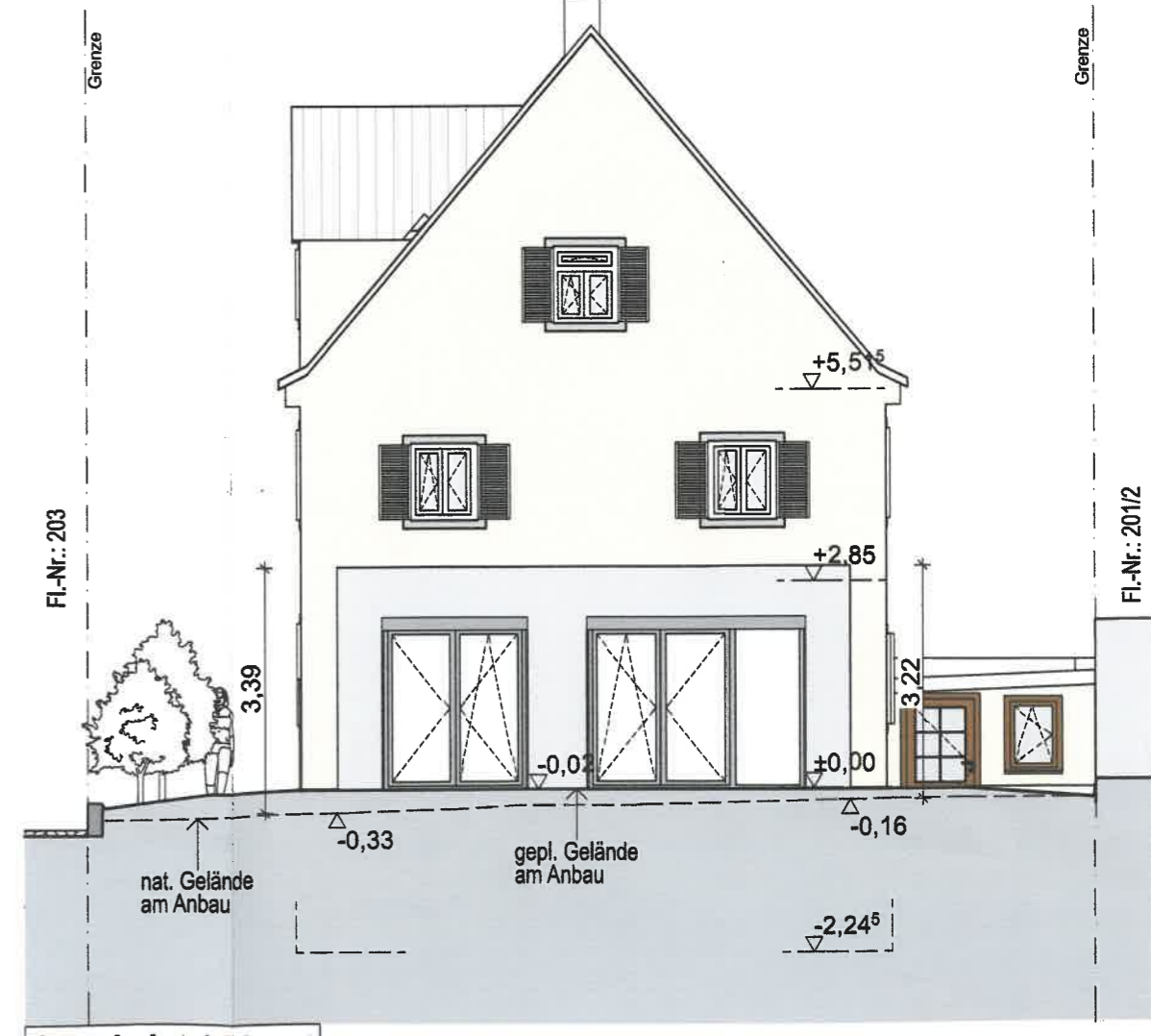
Ansicht West
