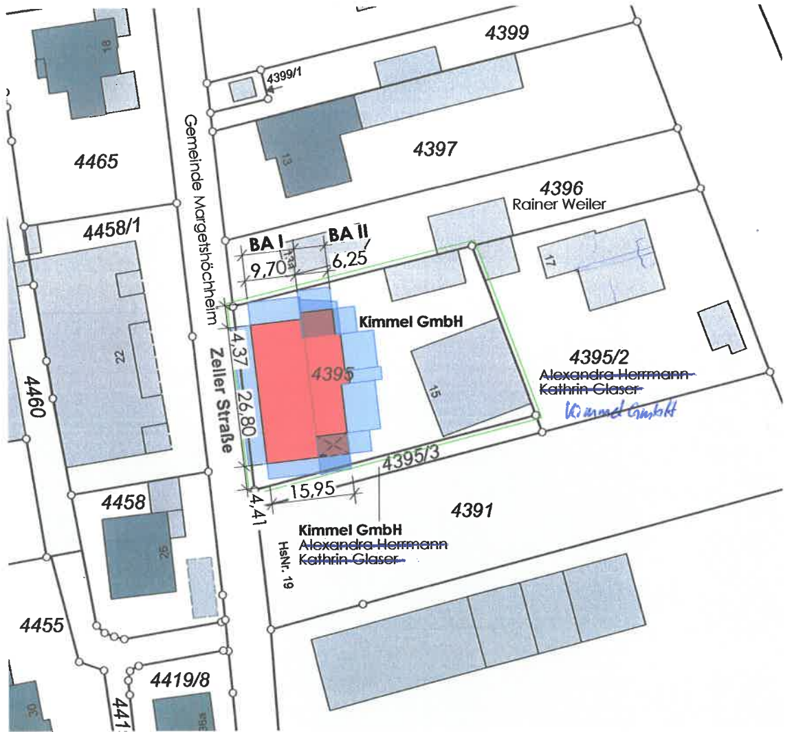
Lageplan, M 1:1000
