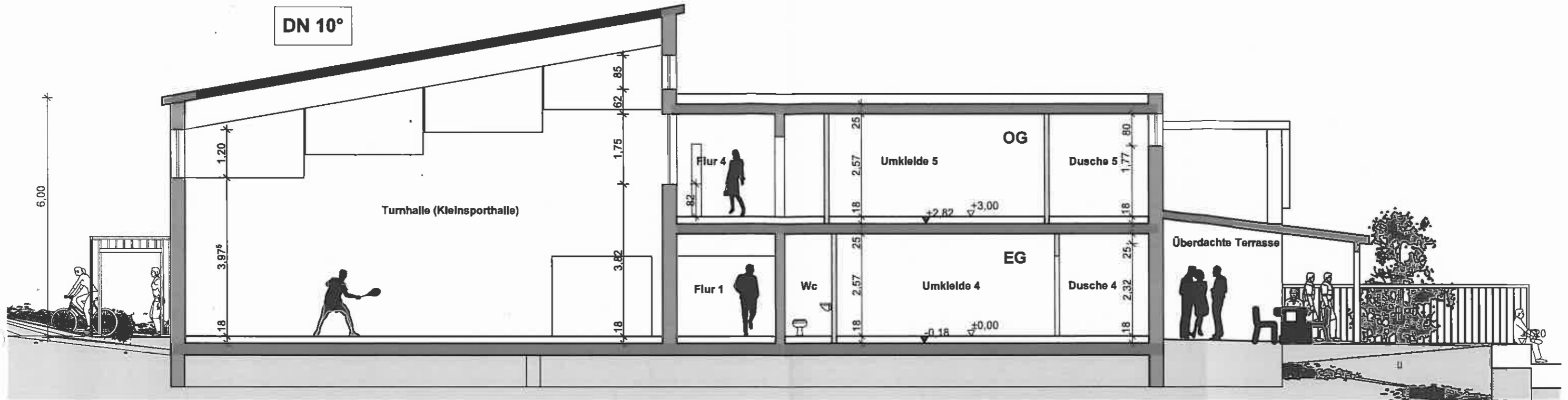
Schnitt A-A
