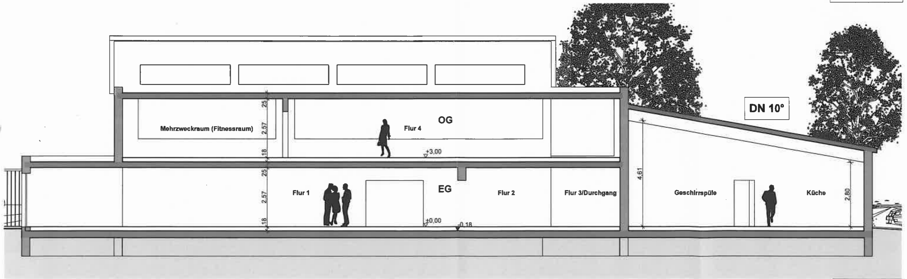
Schnitt B-B
