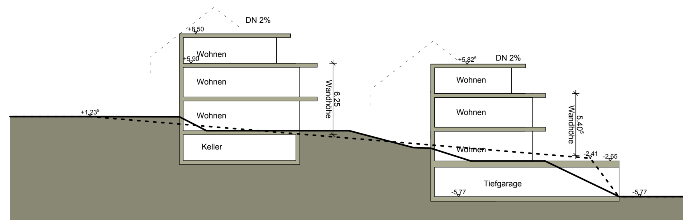
Schemaschnitt
