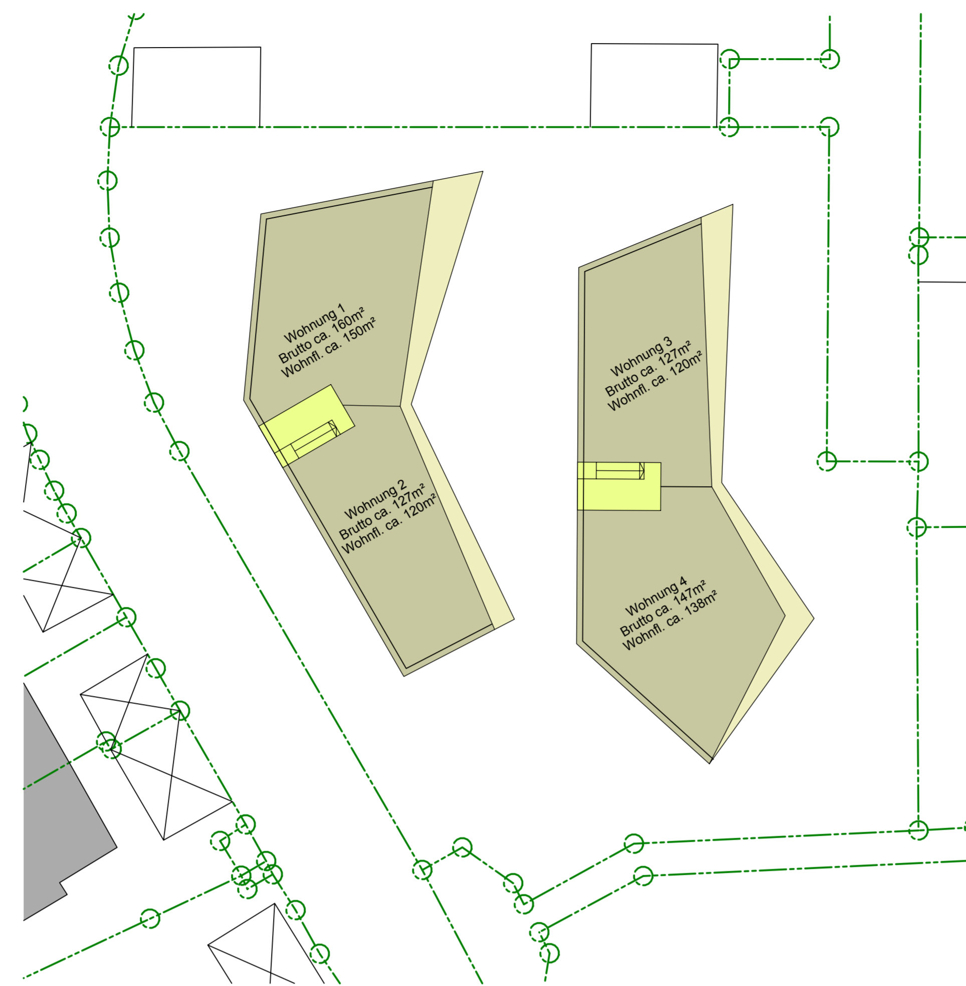
Grundriss Erdgeschoss
