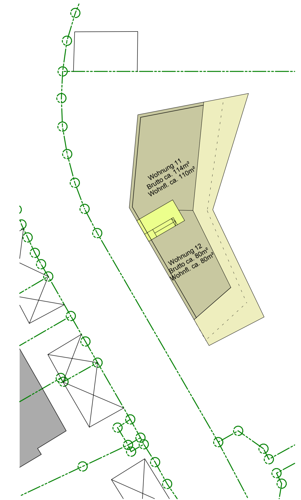
Grundriss Dachgeschoss
