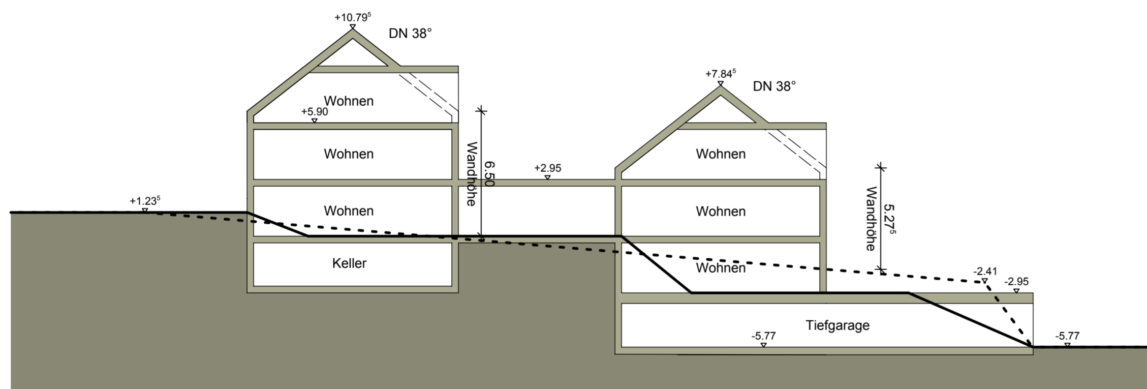
Schemaschnitt
