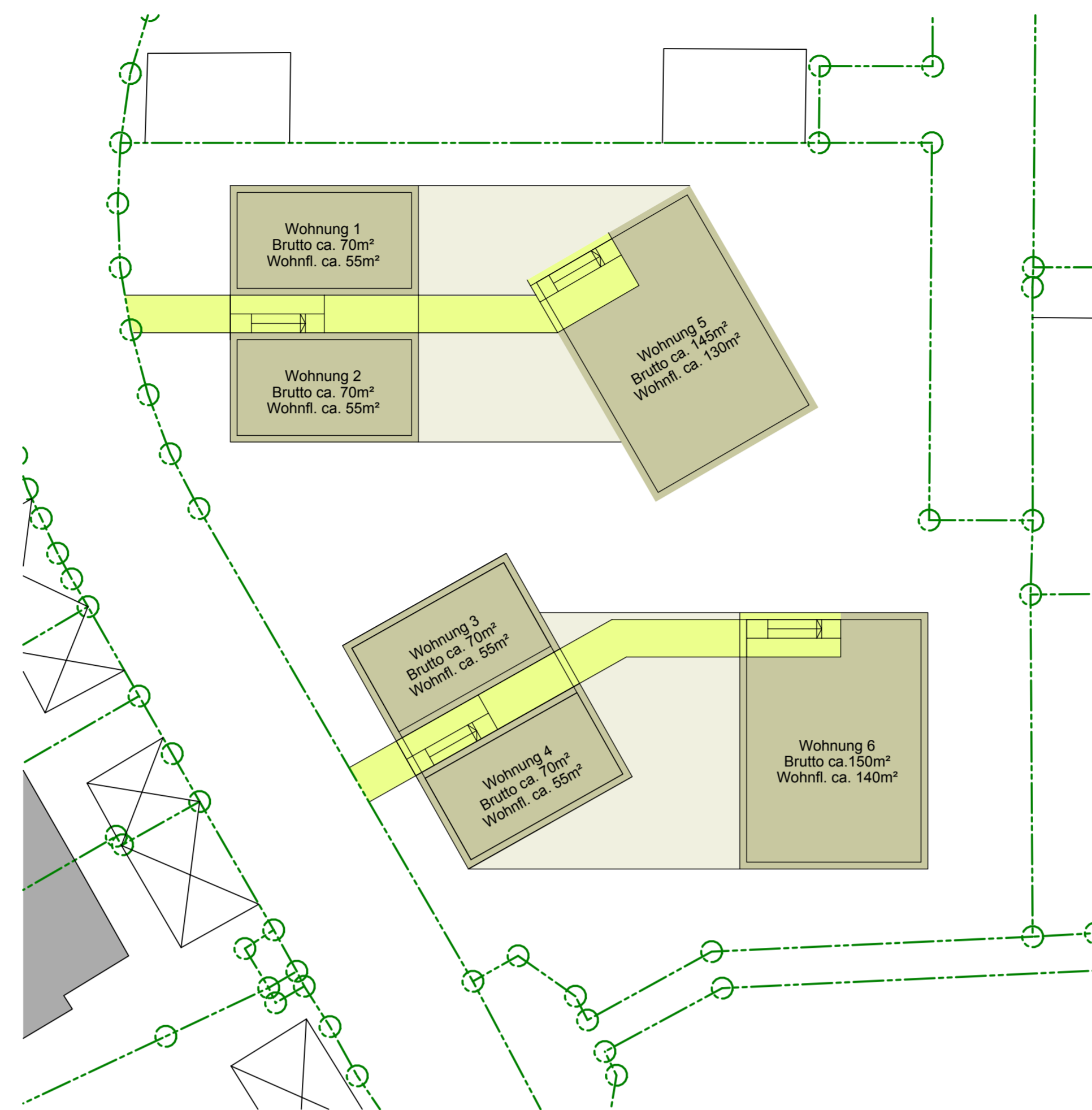
Grundriss Erdgeschoss
